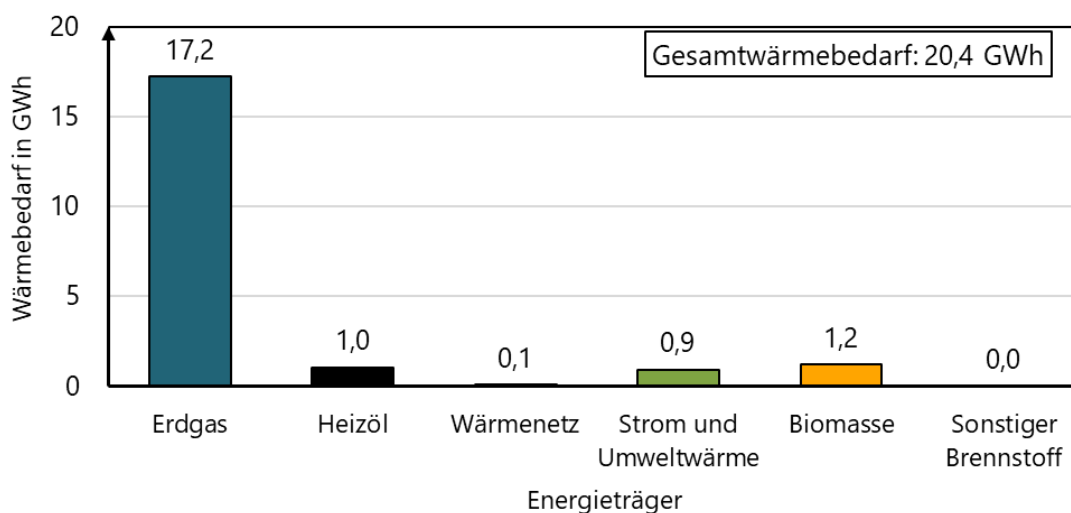
Abbildung 30: Jährlicher Wärmebedarf (Sektor Industrie) in GWh
