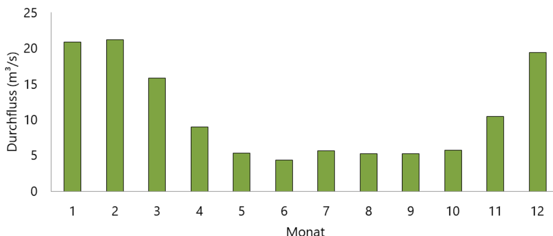
Abbildung 59: Durchschnittlicher monatlicher Durchfluss der Agger (basierend auf Messdaten 2015–2023) [26]
