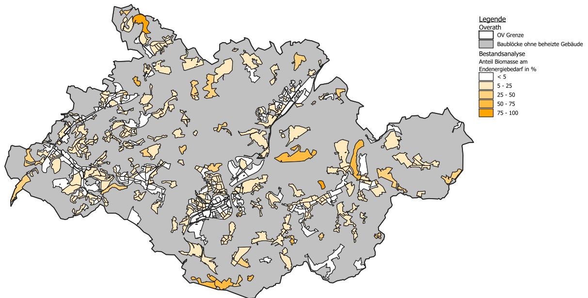
Abbildung 35: Anteil von Biomasse am Wärmebedarf auf Baublockebene
