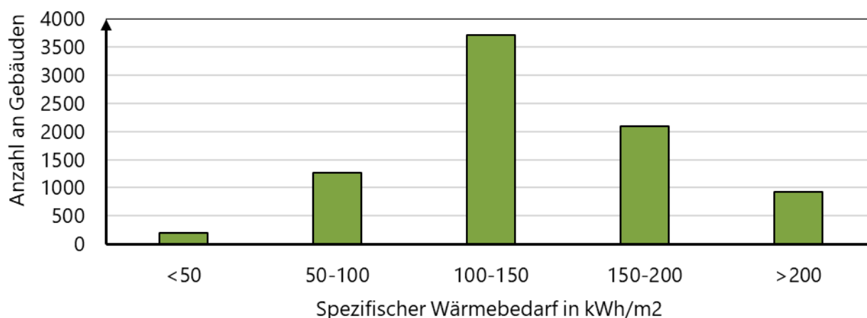
Abbildung 24: Anzahl der Gebäude nach spezifischem Wärmebedarf
