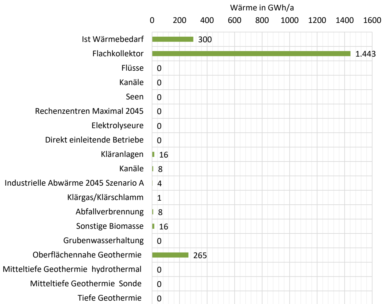
Abbildung 54: Potenziale erneuerbarer Wärmeerzeugung Overath aus der Potenzialstudie zur zukünftigen Wärmeversorgung in NRW [24]
