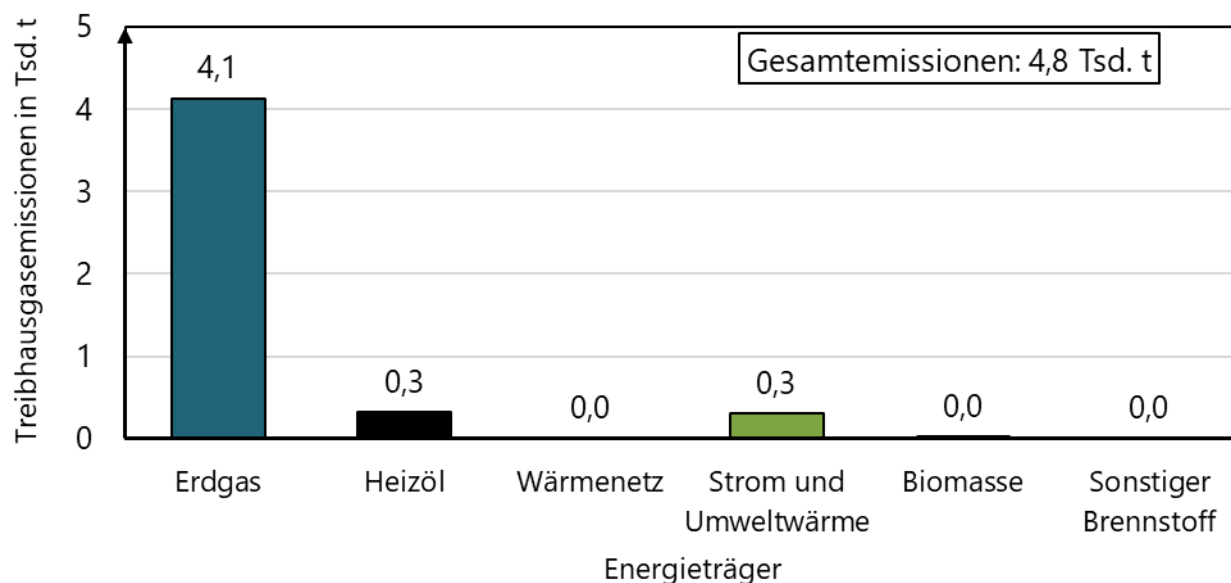
Abbildung 53: Jährliche Treibhausgasemissionen (Sektor Industrie) in Tsd. t
