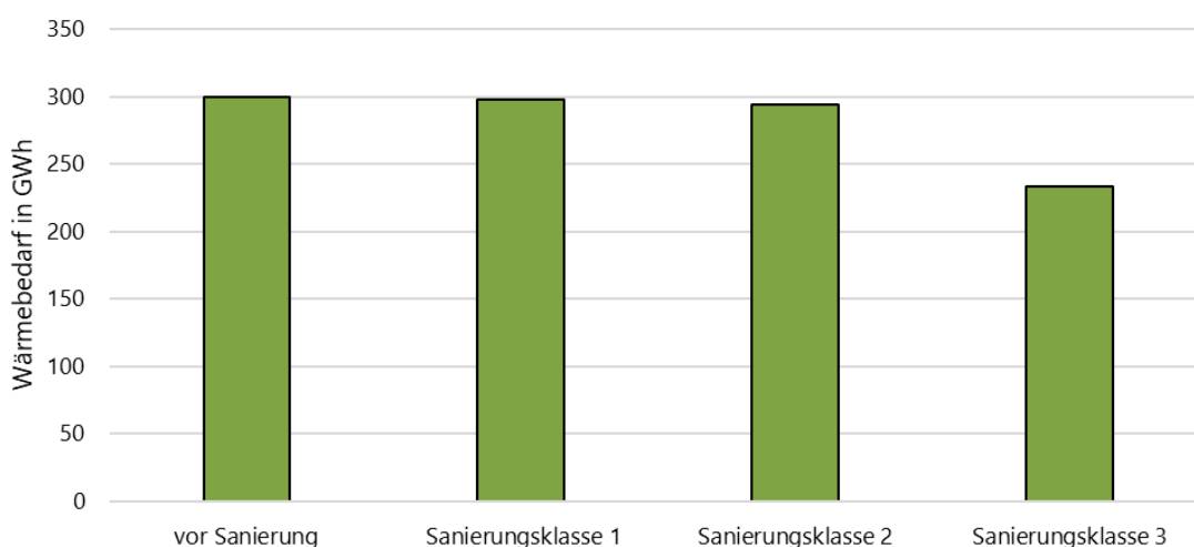
Abbildung 61: Entwicklung des Wärmebedarfs
