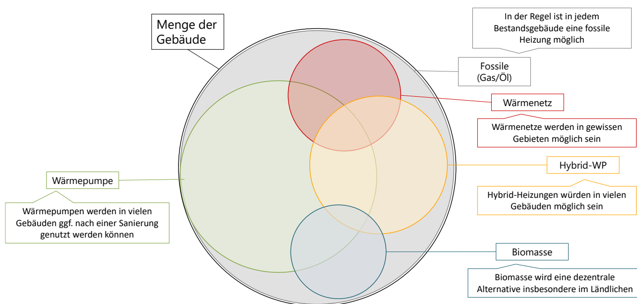
Abbildung 64: Lösungsraum der Wärmetechnologien
