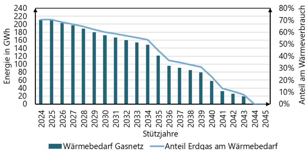
Abbildung 77: Endenergieverbrauch aus Gasnetzen nach Energieträgern und der Anteil der Energieträger am gesamten Endenergieverbrauch der gasförmigen Energieträger
