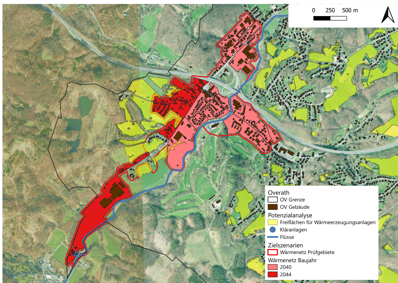
Abbildung 82: Wärmenetz-Prüfgebiet Untereschbach mit Ausbaustufen und Potenzialflächen für Wärmeerzeugung
