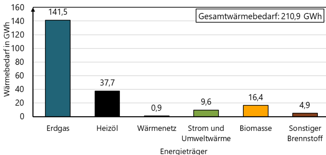
Abbildung 27: Jährlicher Wärmebedarf (Sektor Haushalte) in GWh
