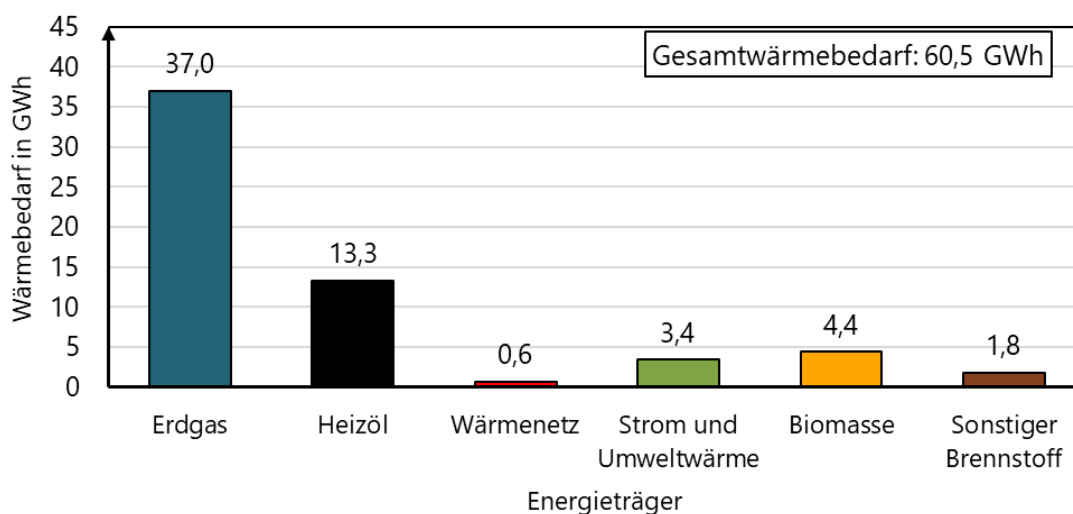
Abbildung 29: Jährlicher Wärmebedarf (Sektor GHD) in GWh
