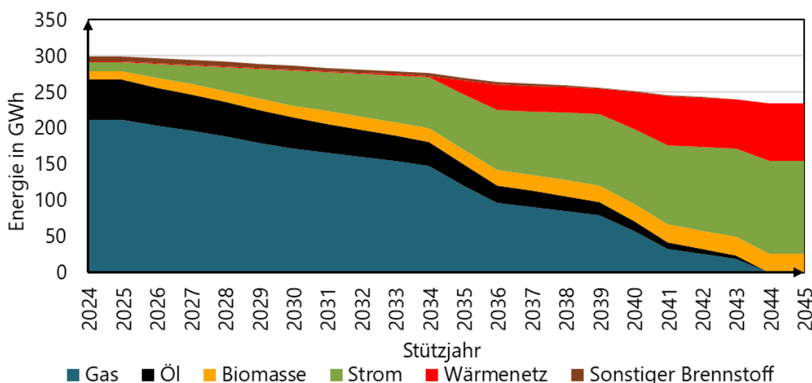
Abbildung 73: Entwicklung Wärmebedarf nach Energieträger
