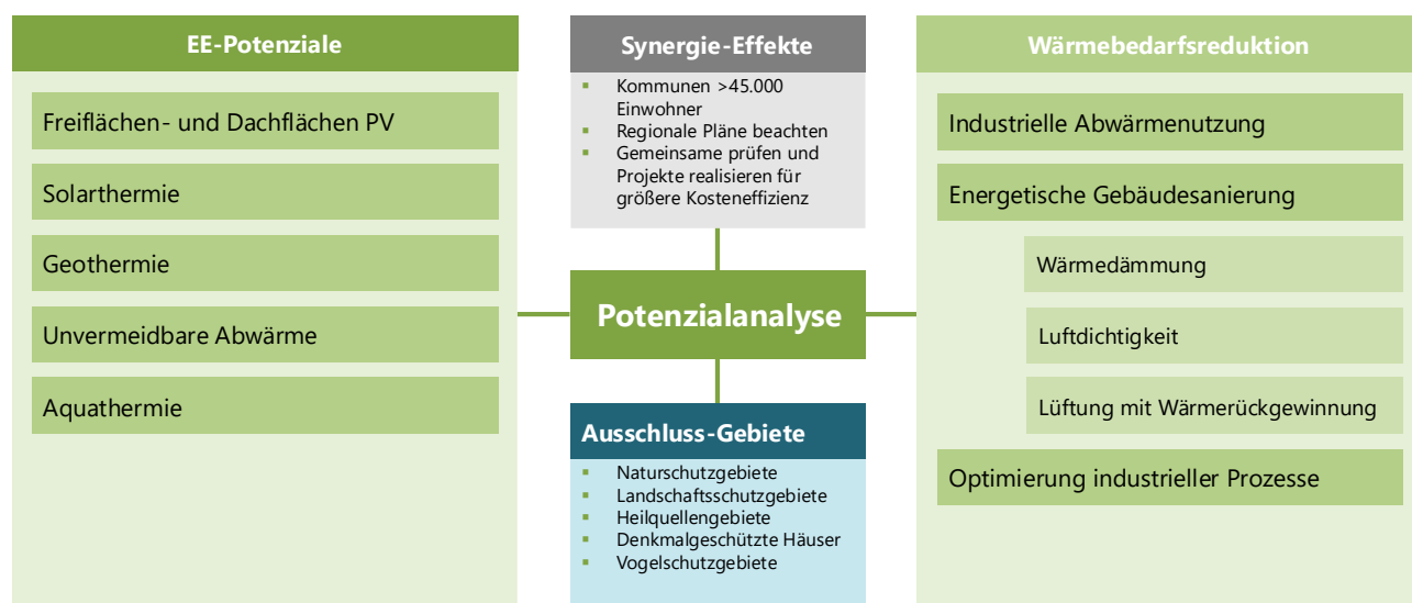
Abbildung 16: EE-Technologien zur Wärmeerzeugung
