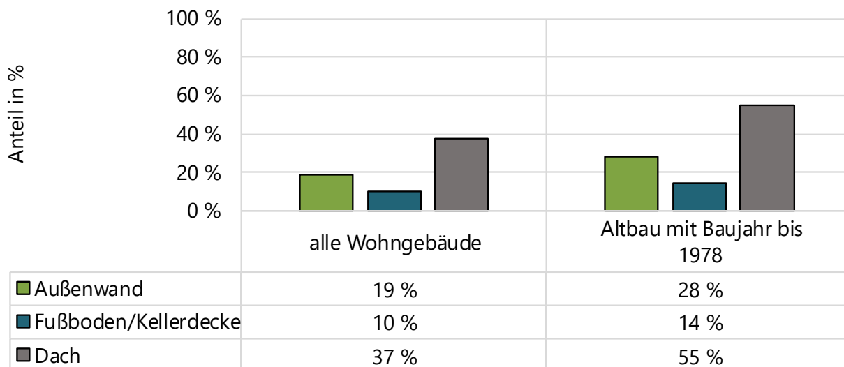
Abbildung 15: Nachträglich gedämmte Bauteilfläche von Außenwänden, Fußböden/Kellerdecken und Dächern (Stand 2016) [13]
