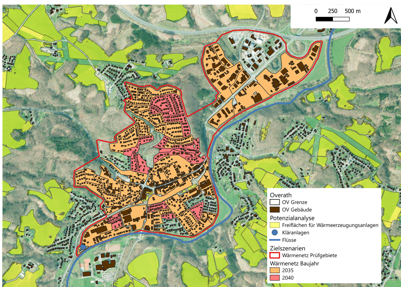
Abbildung 80: Wärmenetz-Prüfgebiet Stadtkern Overath mit Ausbaustufen und Potenzialflächen für Wärmeerzeugung
