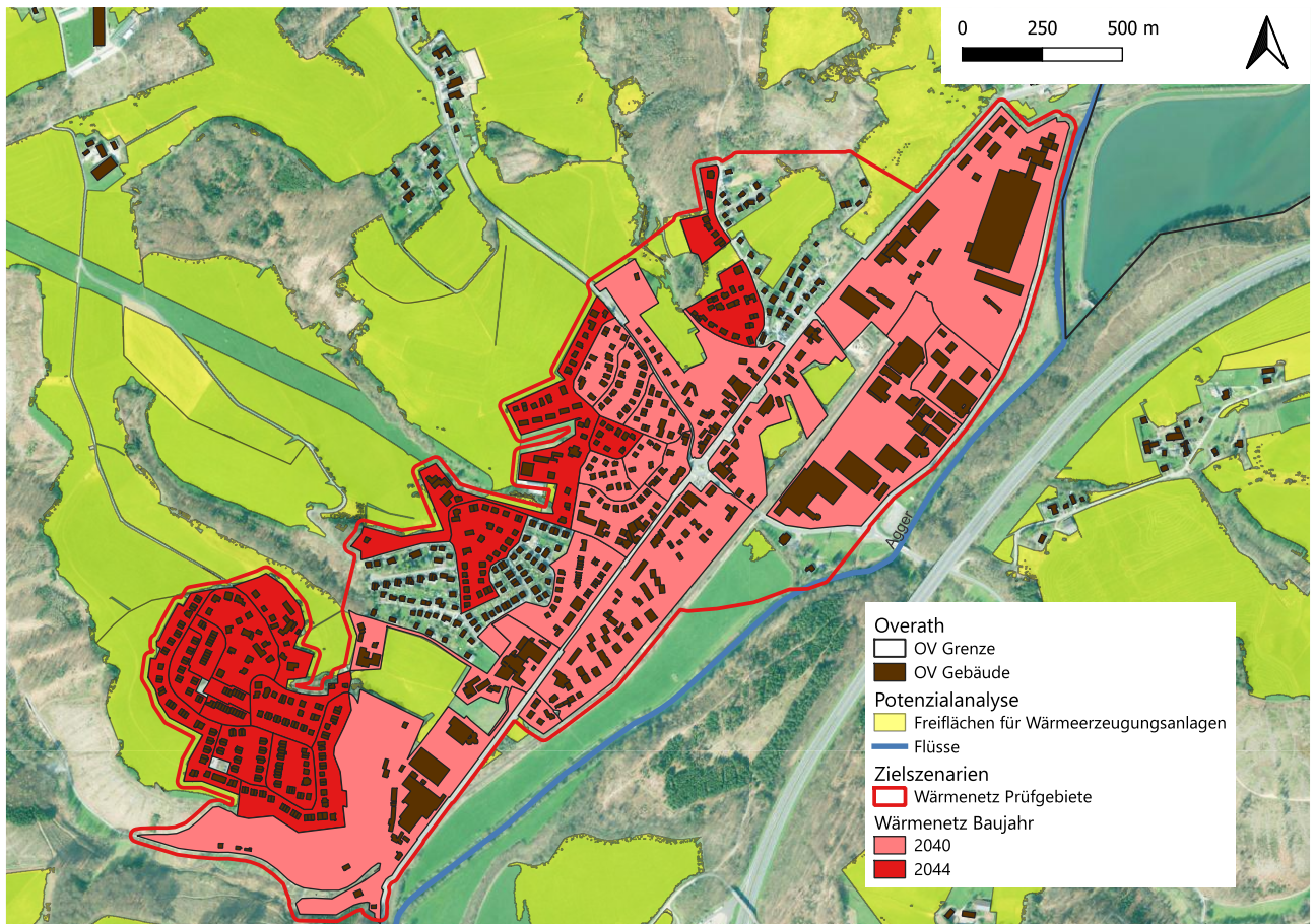
Abbildung 81: Wärmenetz-Prüfgebiet Wilkerath mit Ausbaustufen und Potenzialflächen für Wärmeerzeugung
