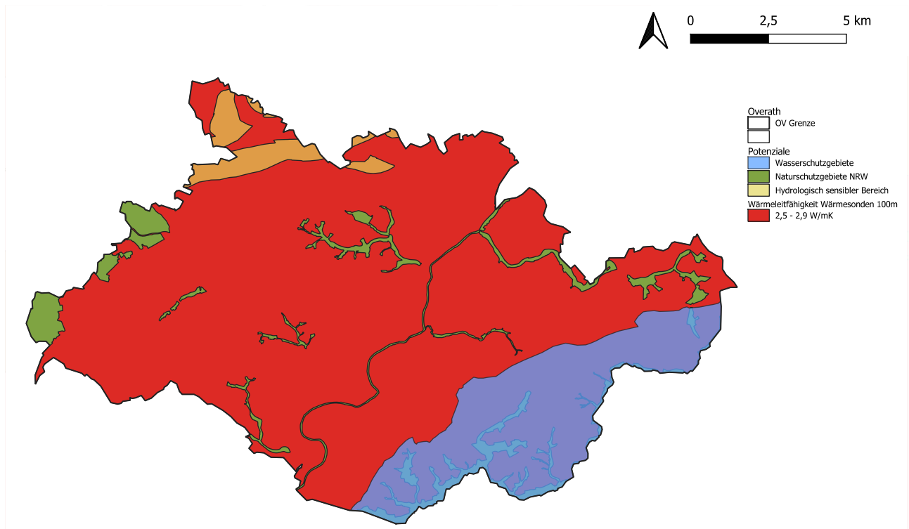
Abbildung 60: Oberflächennahe Geothermie: Ausschlussgebiete und Wärmeleitfähigkeit des Bodens [27]
